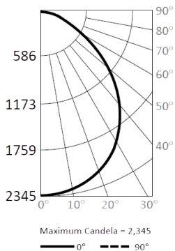
MGRK-B-24X3-44L-QT-40K-CL
