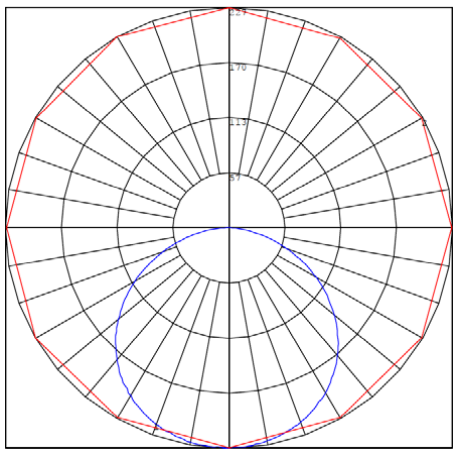
BUG Rating: B2-U1-G0
