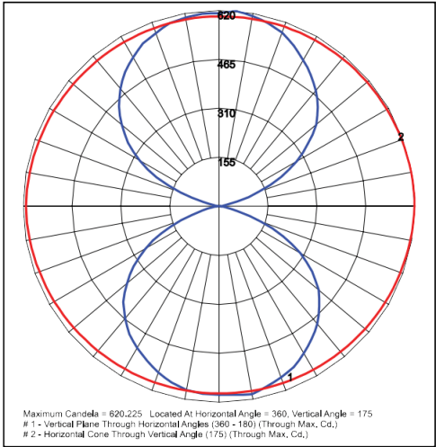
WP31-Q-32L-QT-40K
